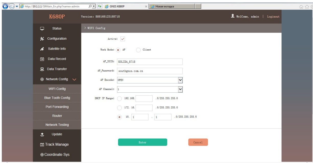
Рисунок 2.3.17 Настройка Сети
